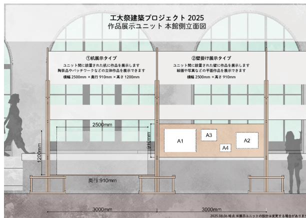
立面図
